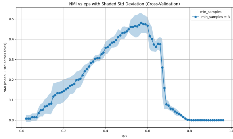
الشكل 27: أثر المعامل \epsilon على النتائج باستخدام mBert لتمثيل الرسائل.
