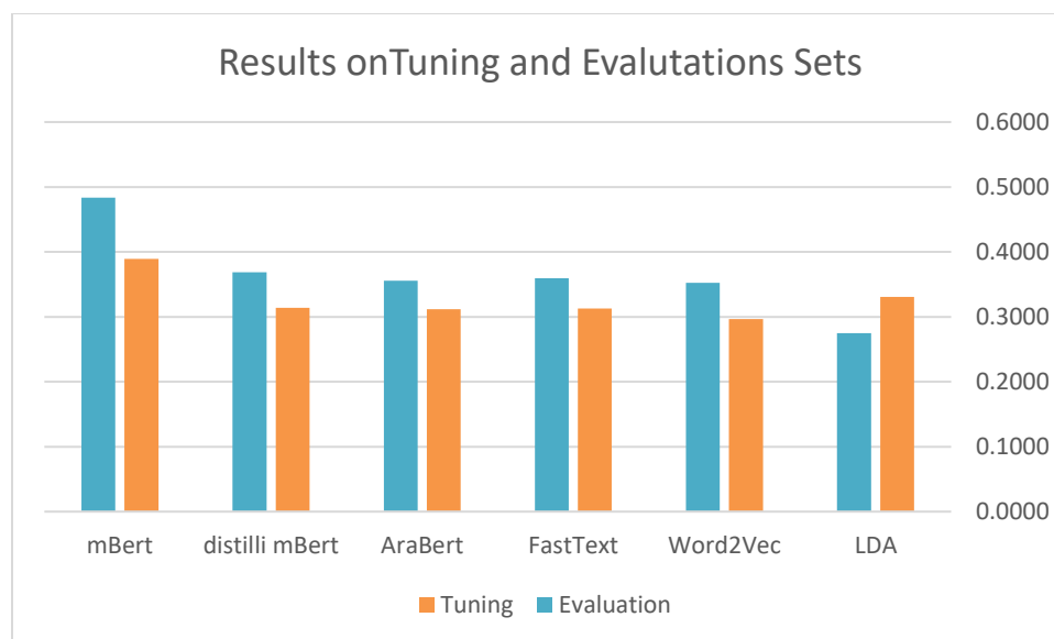
الشكل 31: الفرق بين نتائج الضبط والاختبار.
