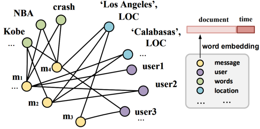
الشكل 3: مثال على شبكة معلومات غير متجانسة.
