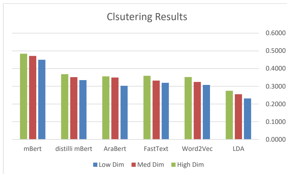
الشكل 30: نتائج العنقدة في التجربة الثانية.
