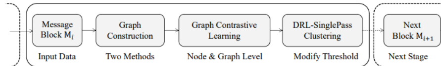
الشكل 7: خط عمل النموذج HCRC.
