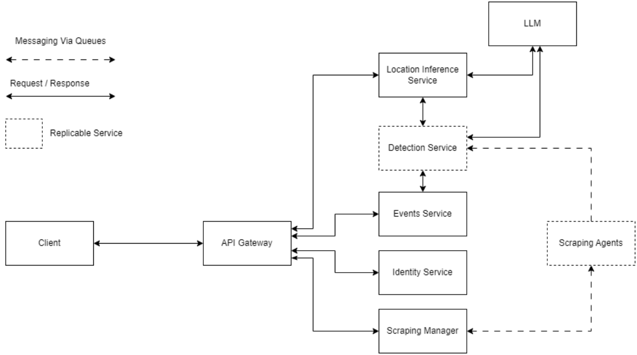
الشكل 14: مخطط خدمات النظام التصميمي.
