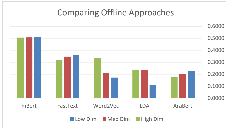
الشكل 28: نتائج التجربة الأولى.
