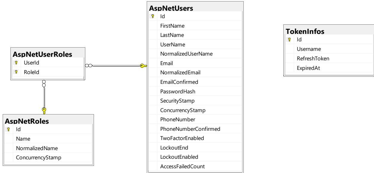
الشكل 56: مخطط قاعدة المعطيات لخدمة الهوية.
