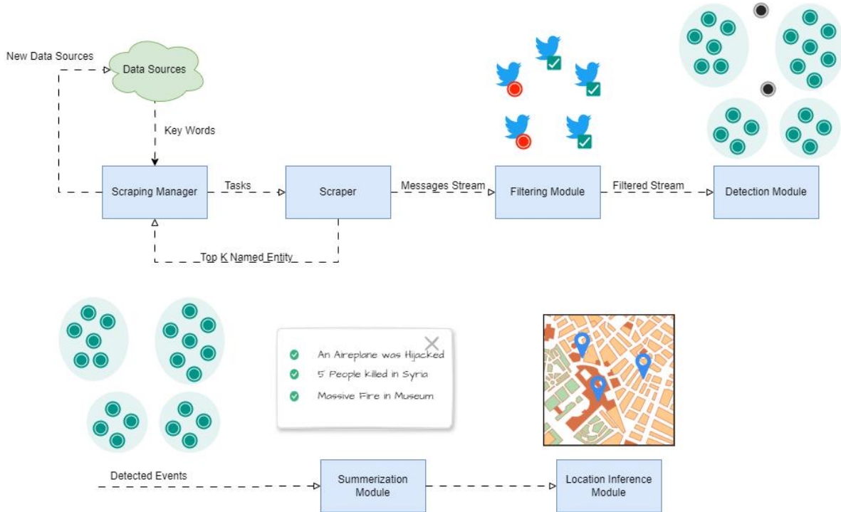
الشكل 11: البنية العامة للمنهجية.
