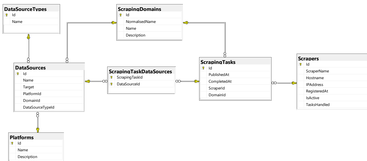
الشكل 45: مخطط قاعدة المعطيات الخاص بخدمة إدارة عمليات سحب البيانات.
