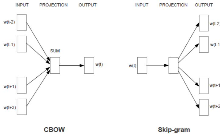
الشكل 2: نموذج Skip Gram و CBOW.
