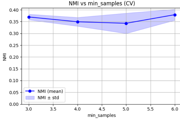
الشكل 29: أثر معامل حجم العينات على النتائج.
